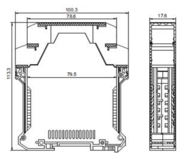
【安装尺寸】
