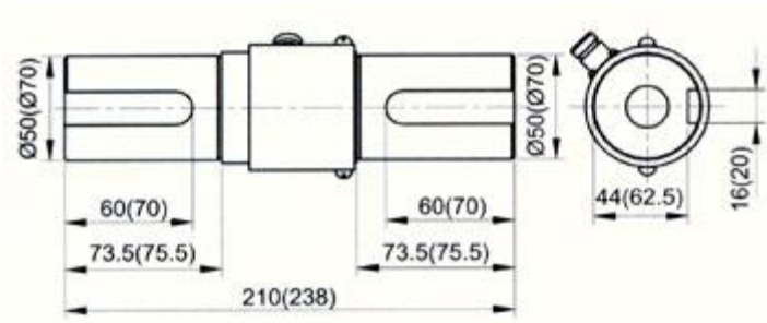
注：括号内尺寸为AKC-17C型
