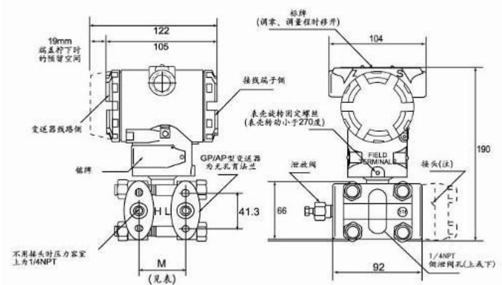
外形尺寸图
